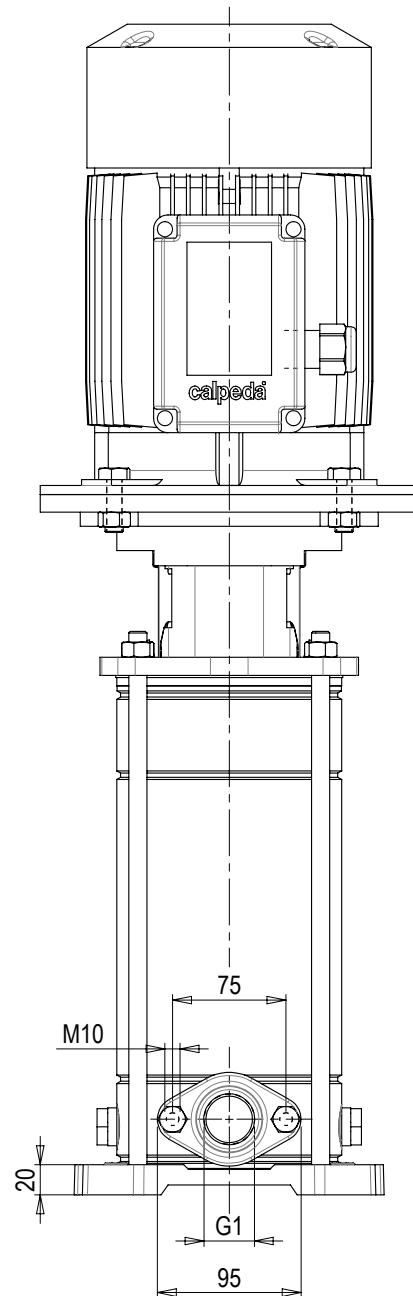
SEZ. A-A
