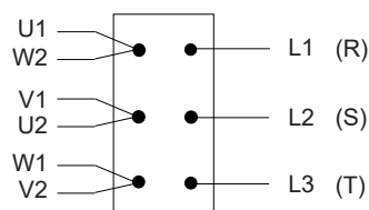
Schalttafelanschluss
