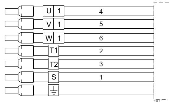
Identificazione conduttori cavo elettropompe
