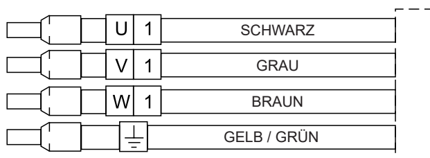
Identifizierung der Leiter der Elektropumpenkabel
