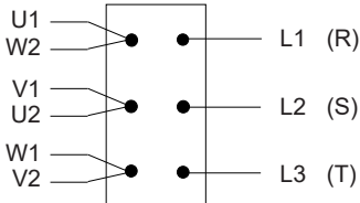
Branchement tableau
