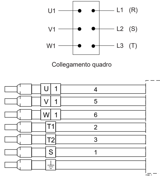
Identificazione conduttori cavo elettropompe
