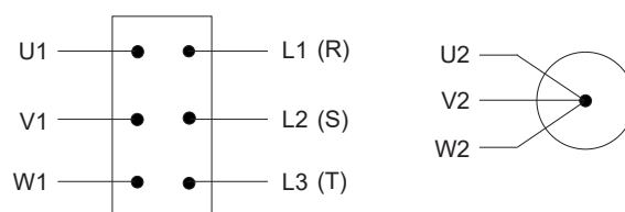
Collegamento quadro
