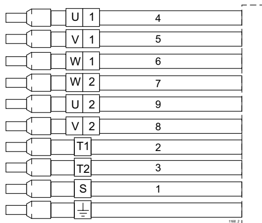
Σύνδεση πίνακα
