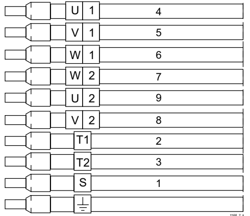
Identifizierung der Leiter der Elektropumpenkabel
