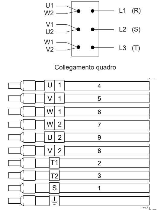
Identificazione conduttori cavo elettropompe
