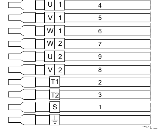
Identificazione conduttori cavo elettropompe
