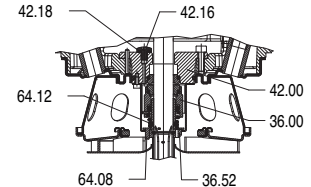
VERSIONE TENUTA BILANCIATA
