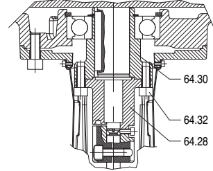
VERSIONE MEC132 - MEC160
