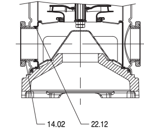
VERSIONE CAMICIA CON FLANGE OVALI
